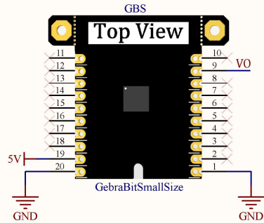
GEBRABIT PINOUT
