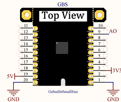
GEBRABIT PINOUT
