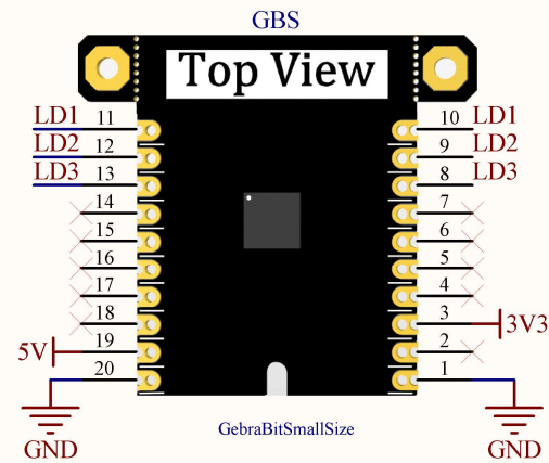
GEBRABIT PINOUT
